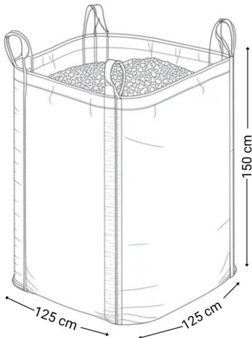
Rysunek 1. Orientacyjne wymiary napełnionego worka Big-Bag (1,5 m 3 )
